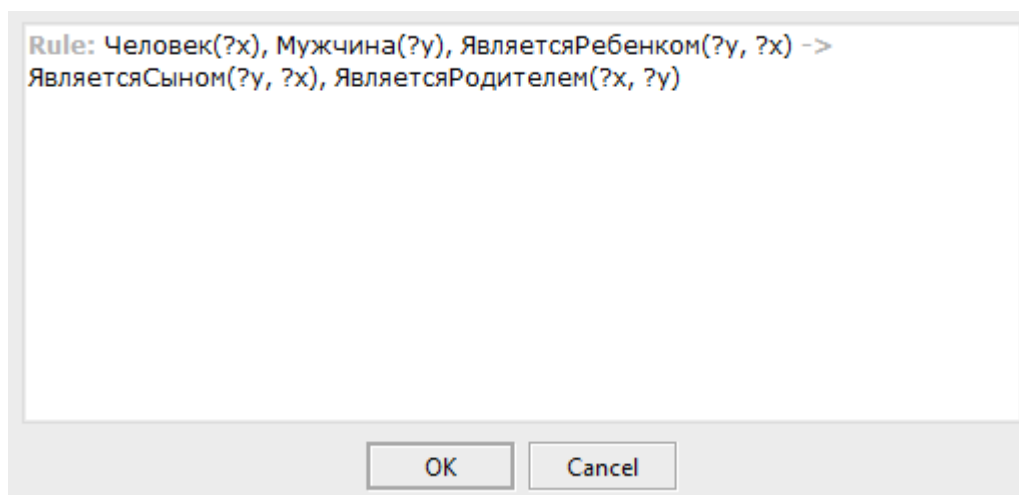
Рис. 28. Создание правила SWRL в редакторе Protégé 5.
