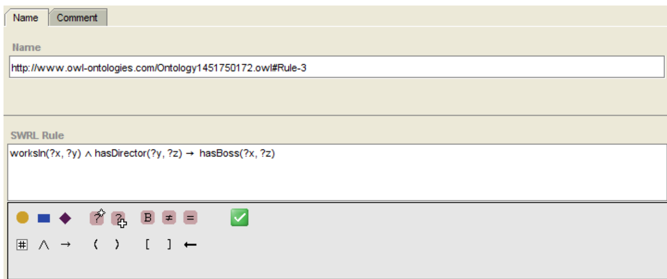
Рис. 27. Создание SWRL-правила в редакторе Protégé 3.
