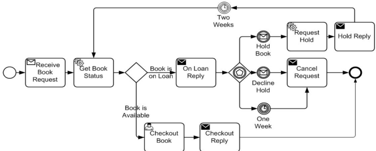
Фигура 10.1 – Пример Процессы
