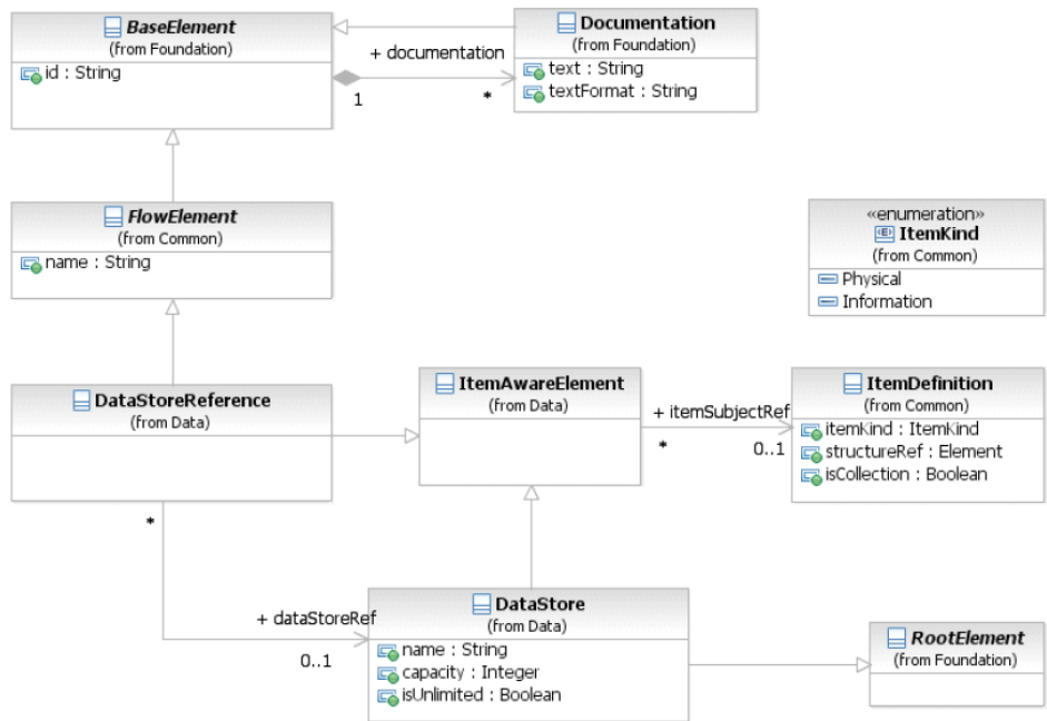
Фигура 10.55 – Диаграмма классов элемента DataStore
