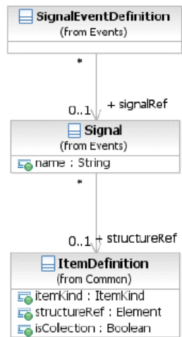
Фигура 10.93 - Диаграмма классов элемента SignalEventDefinition
