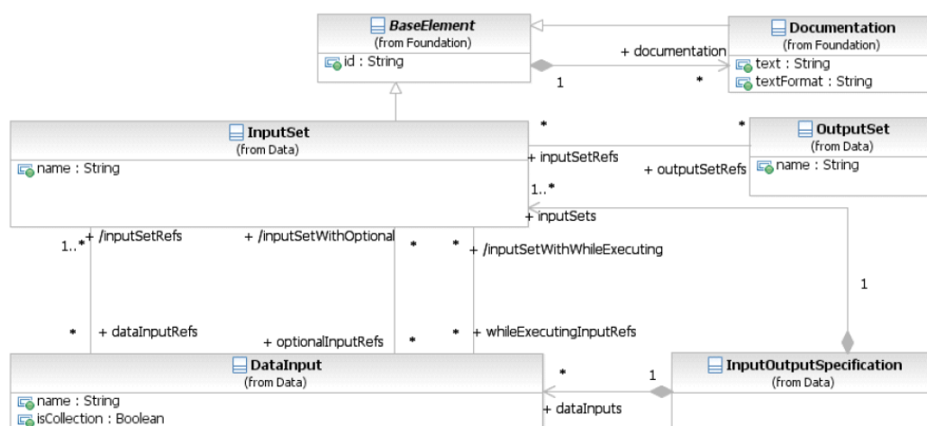
Фигура 10.62 – Диаграмма классов элемента InputSet
