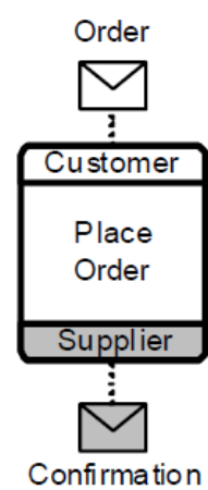
Фигура 8.29 – Сообщения, графически ассоциированные с Задачей Хореографии
