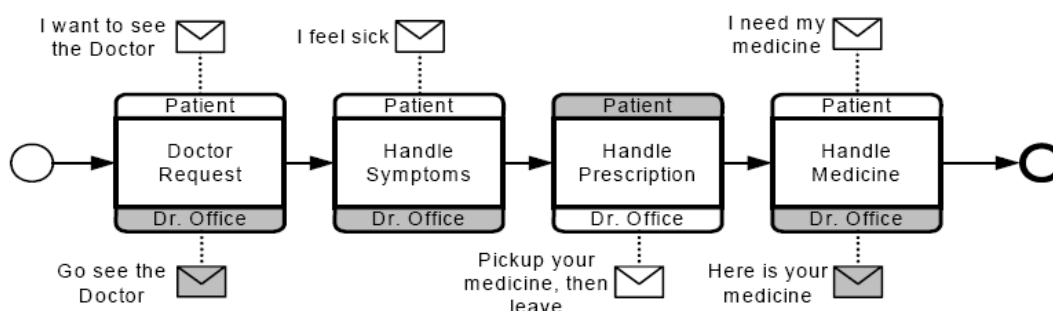
Фигура 7.4 – пример Хореографии
