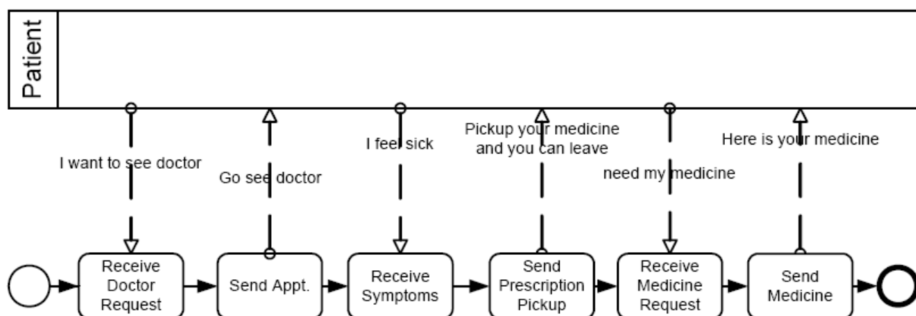
Фигура 7.2 – Пример публичного Процесса
