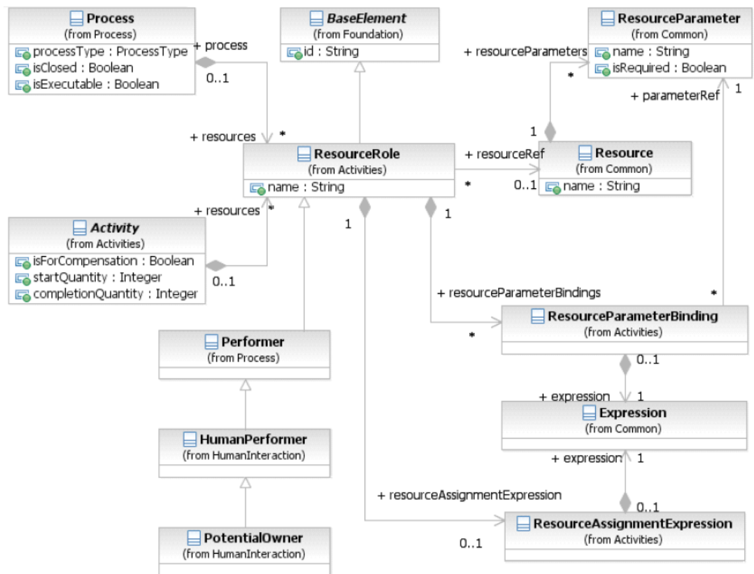
Фигура 10.7 – Диаграмма классов для распределения ресурсов
