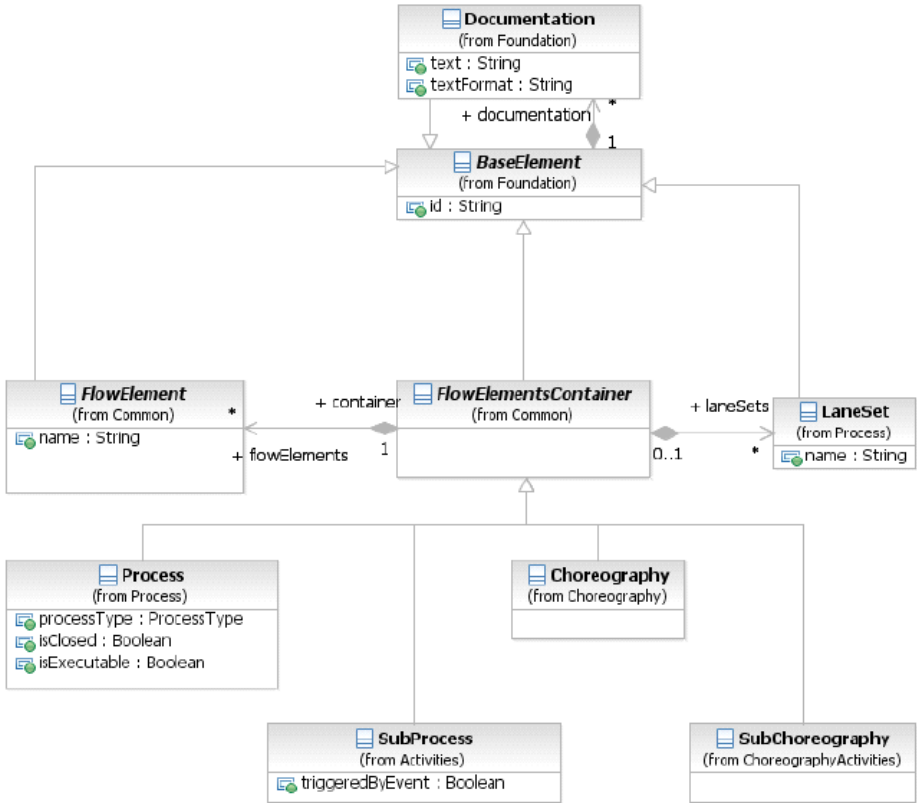
Фигура 8.23 – Диаграмма классов элемента FlowElementContainers
