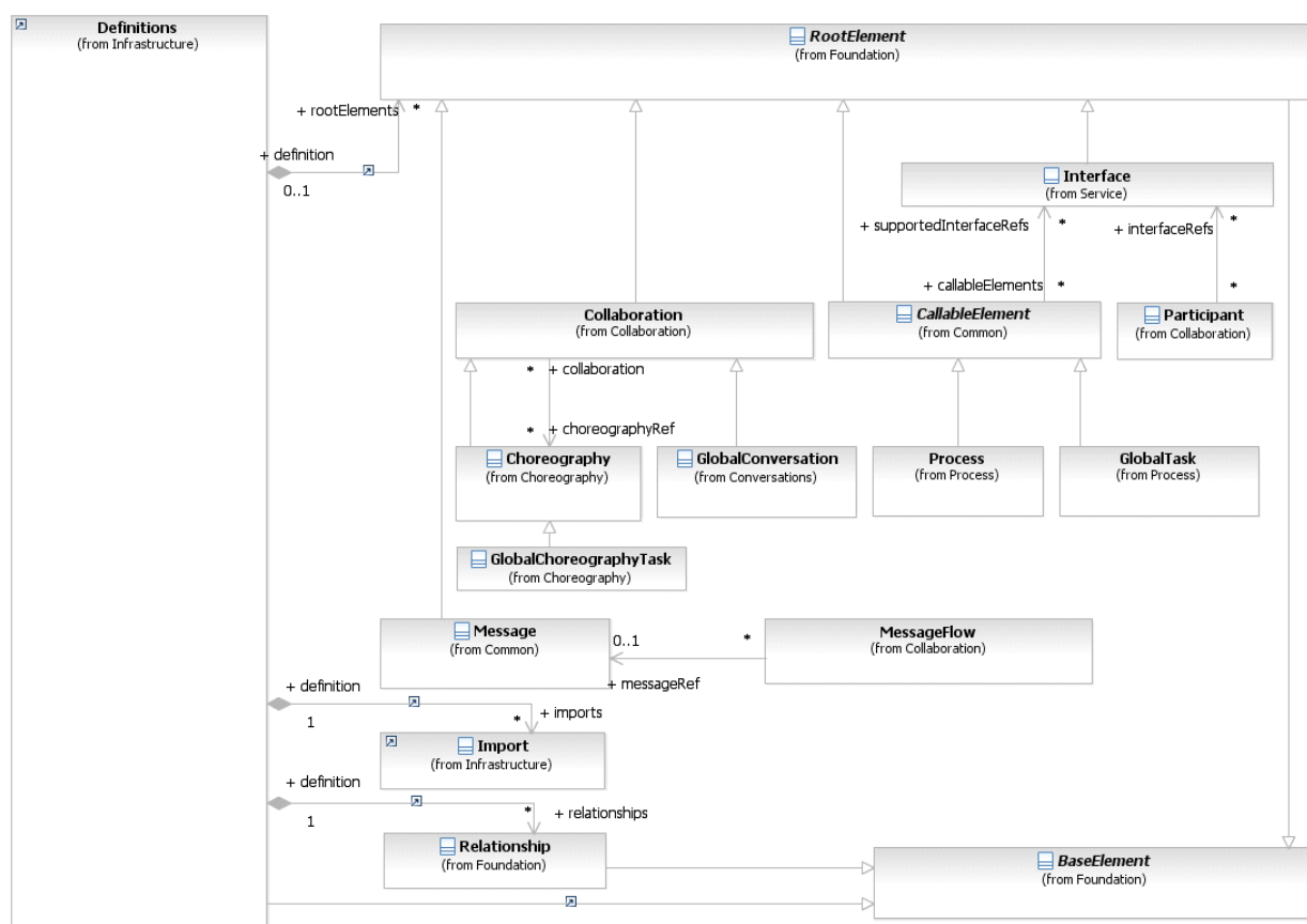
Фигура 8.3 – Диаграмма классов, отображающая организацию основных элементов ВРМН
