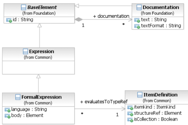
Фигура 8.21 – Диаграмма классов элемента Expression
