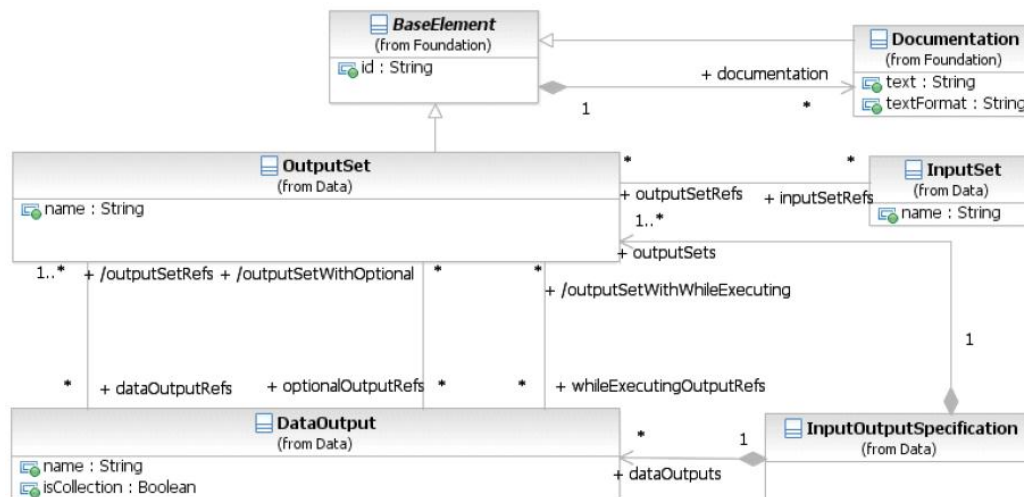
Фигура 10.63 – Диаграмма классов элемента OutputSet
