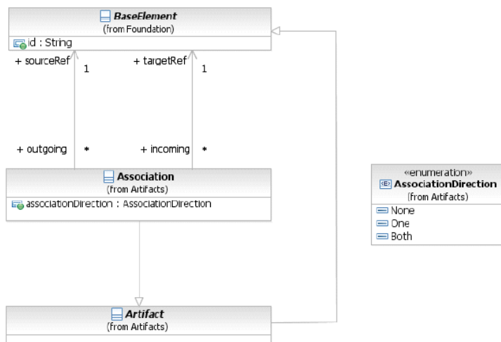
Фигура 8.10 – Диаграмма класса Association
