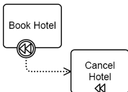
Фигура 10.121 – Компенсация, использующая Событие на границе Действия
