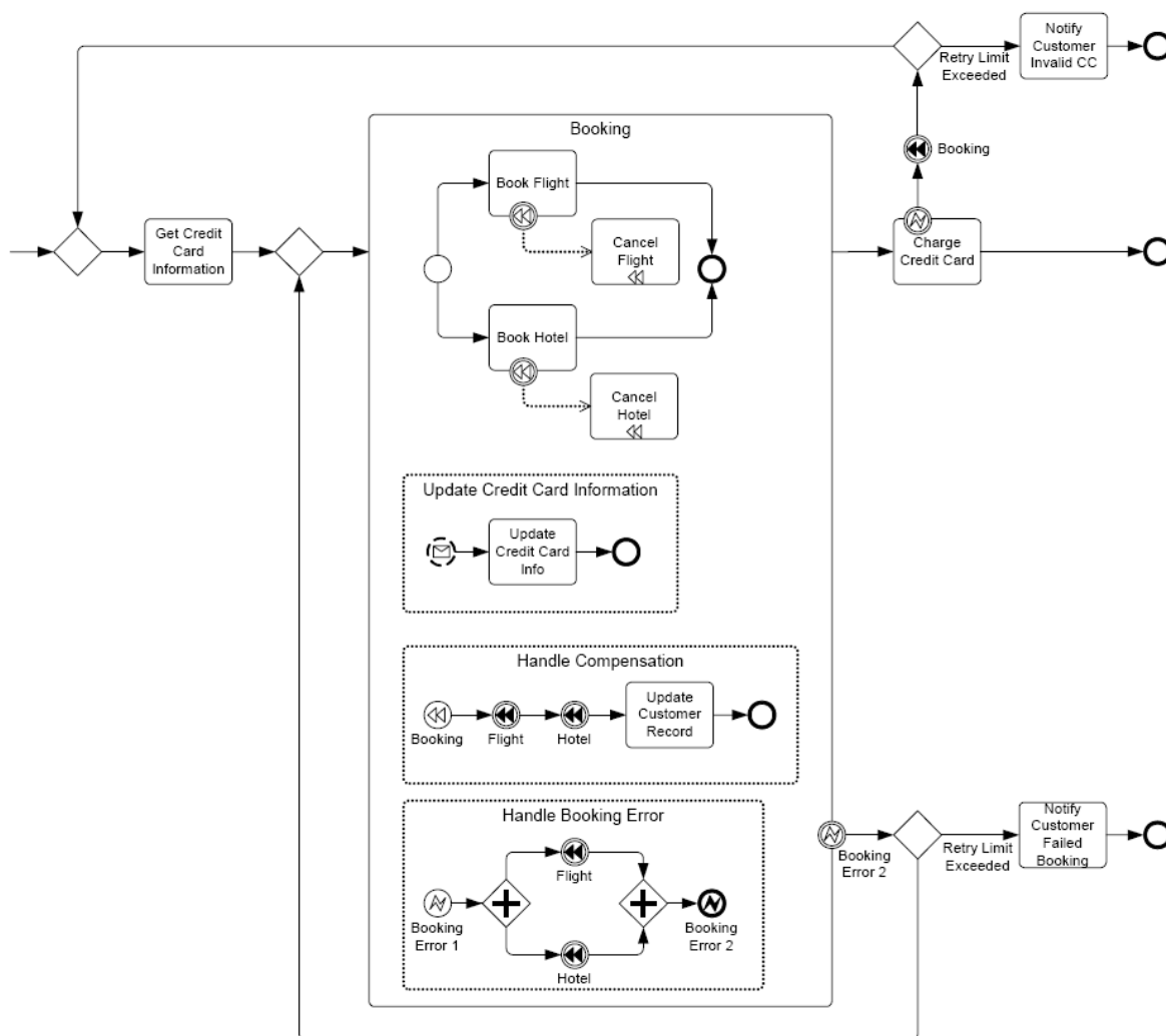
Фигура 10.100 – Пример Процесса, содержащего работающие Событийные Подпроцессы для встроенной обработки Событий
