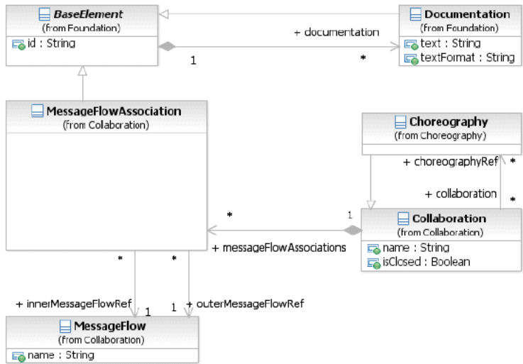
Фигура 9.15 – Диаграмма классов элемента MessageFlowAssociation
